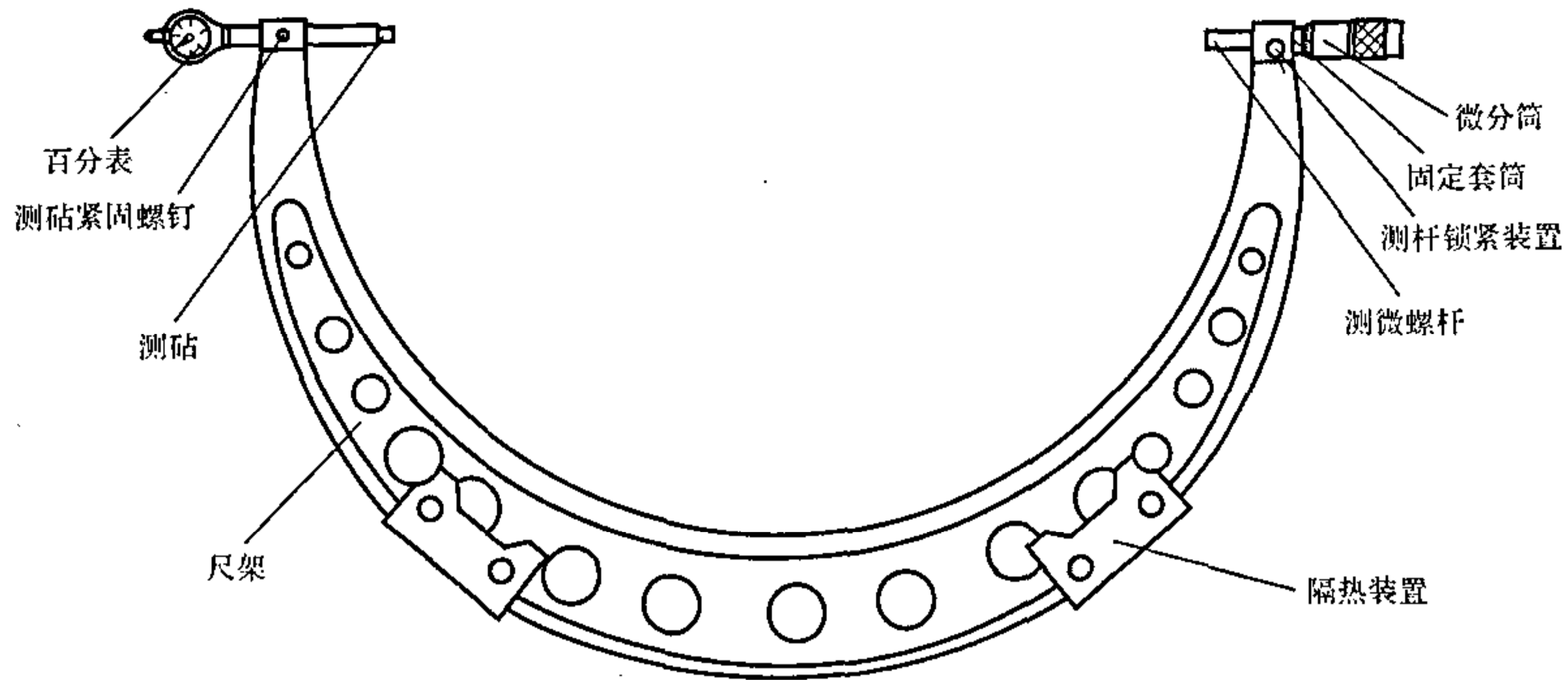
图2 测砧带表式外径千分尺
