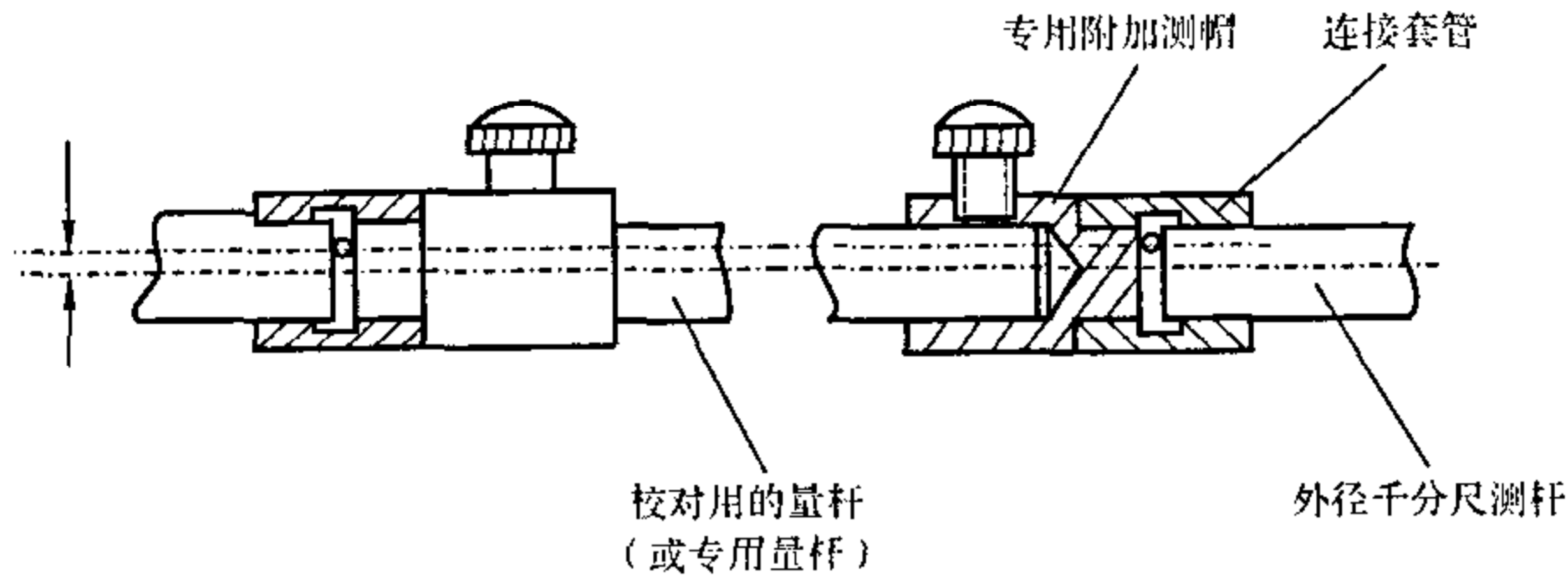
图 5 钢球式专用检具
