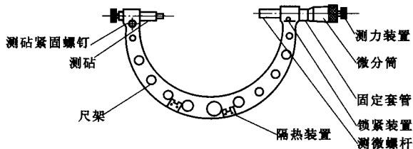
图 2 测砧为可换式或可调式的千分尺
