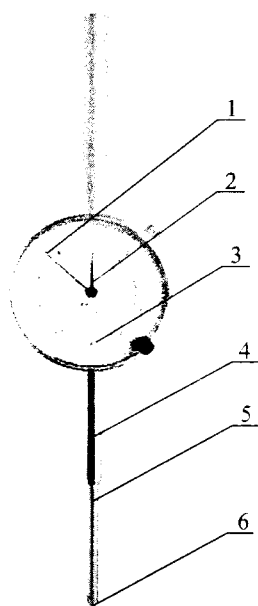
图 1 指针式百分表
