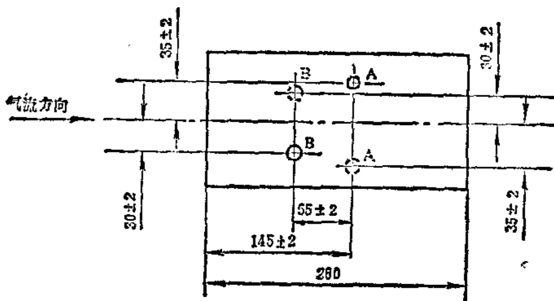
皮托管安装孔 (A) 与风速表安装 孔 (B) 在工作段底板上的位置示意图
