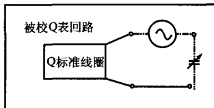
图4 Q表Q值校准连接示意图
