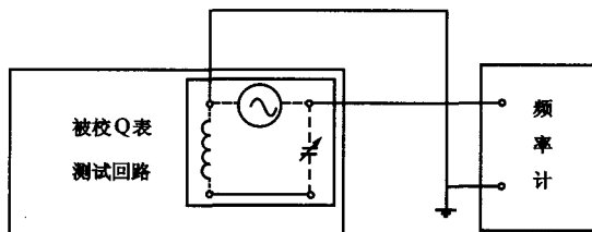
图3 Q表信号源频率刻度校准
