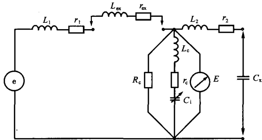
图 B1 Q 表测试回路等效电路
