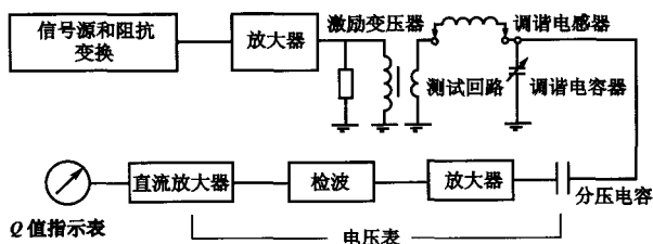
图1 典型Q表框图
