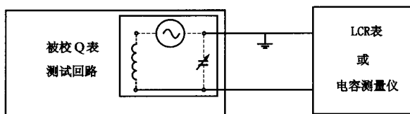
图 2 Q 表电容刻度校准连接框图
