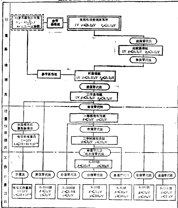
直流电动势计量器具检定系统框图
