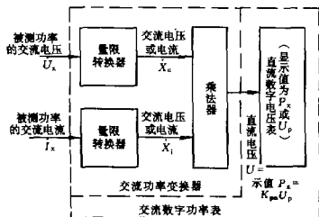
图 1 交流数字功率表的测量框图
